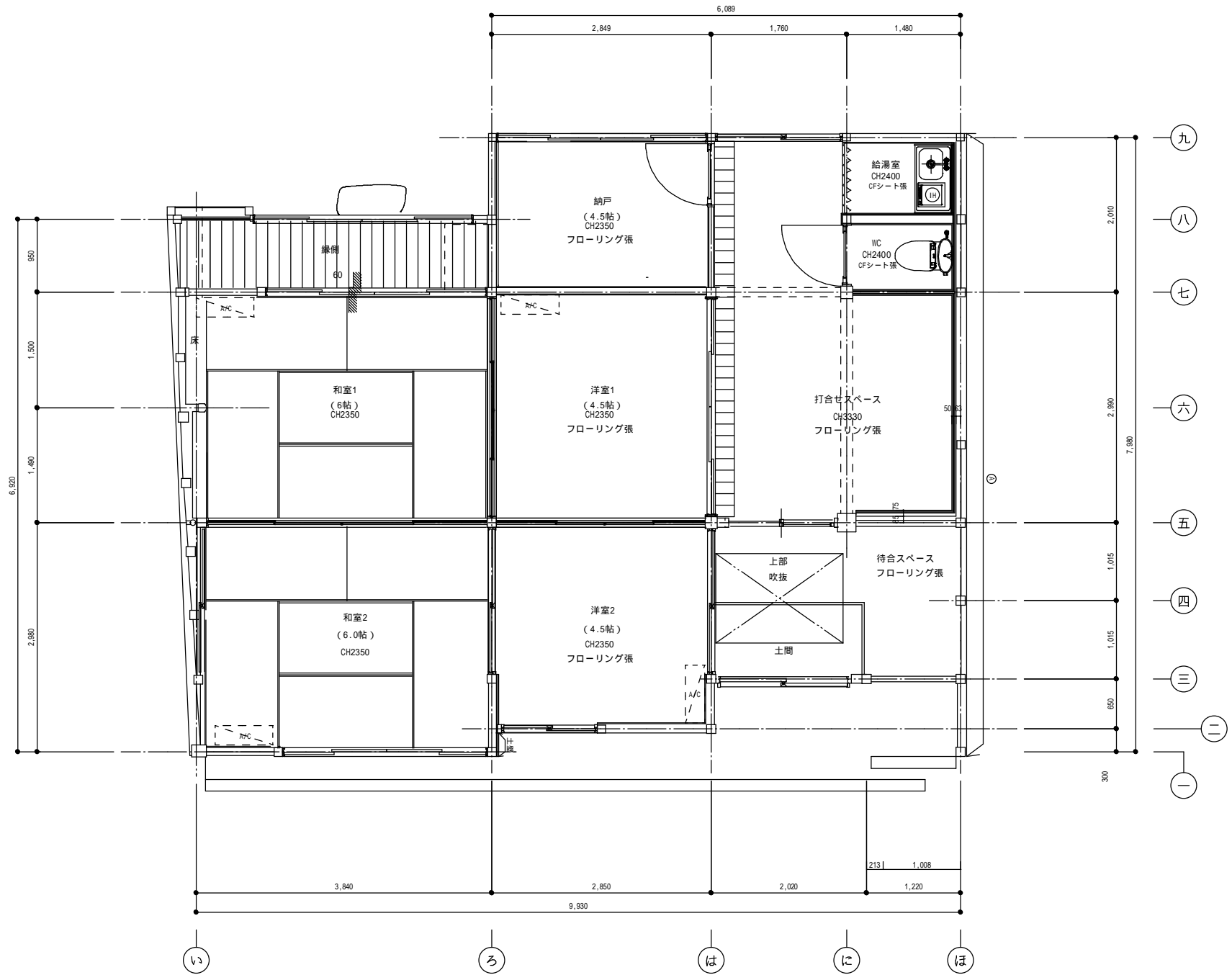
オフィス用途での母屋改修計画平面図
