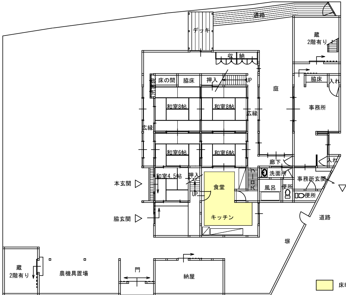
1階 平面図
