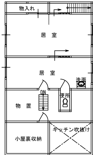
2階 平面図
