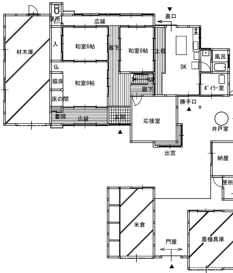
1階 平面図
